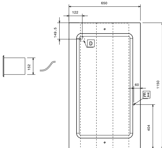
Boven aanzicht
